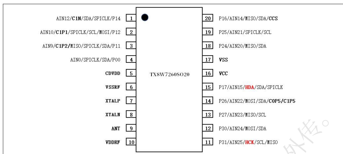
图 2 - TX8W7260S020 (SOP20) 封装图
