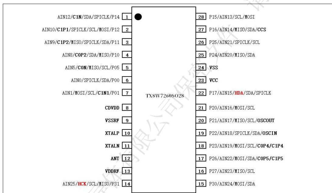
图 3 - TX8W7260S028 (SOP28) 封装图
