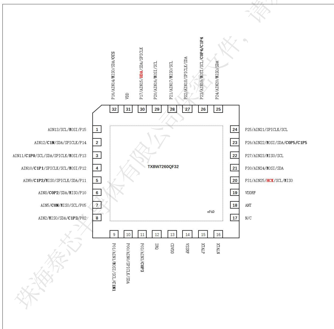
图 1 - TX8W7260QF32 (QFN32) 封装图
